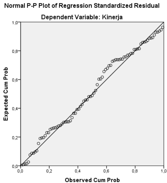
Gambar 3 Uji Normalitas
